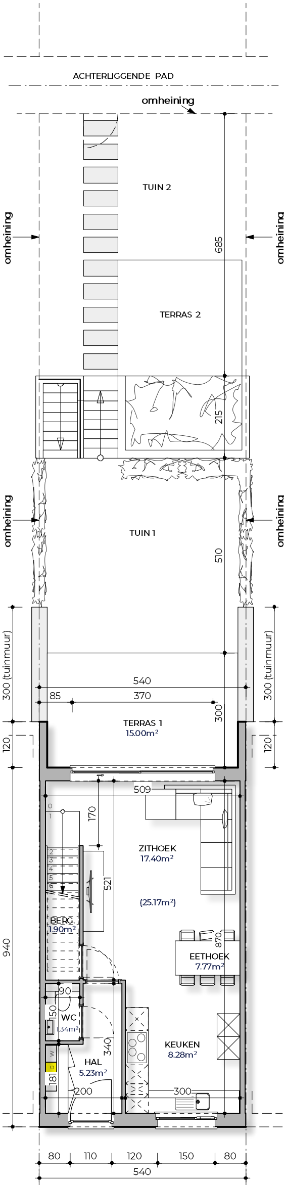
GRONDPLAN - schaal 1/100 bruto-oppervlakte: 51m 2
